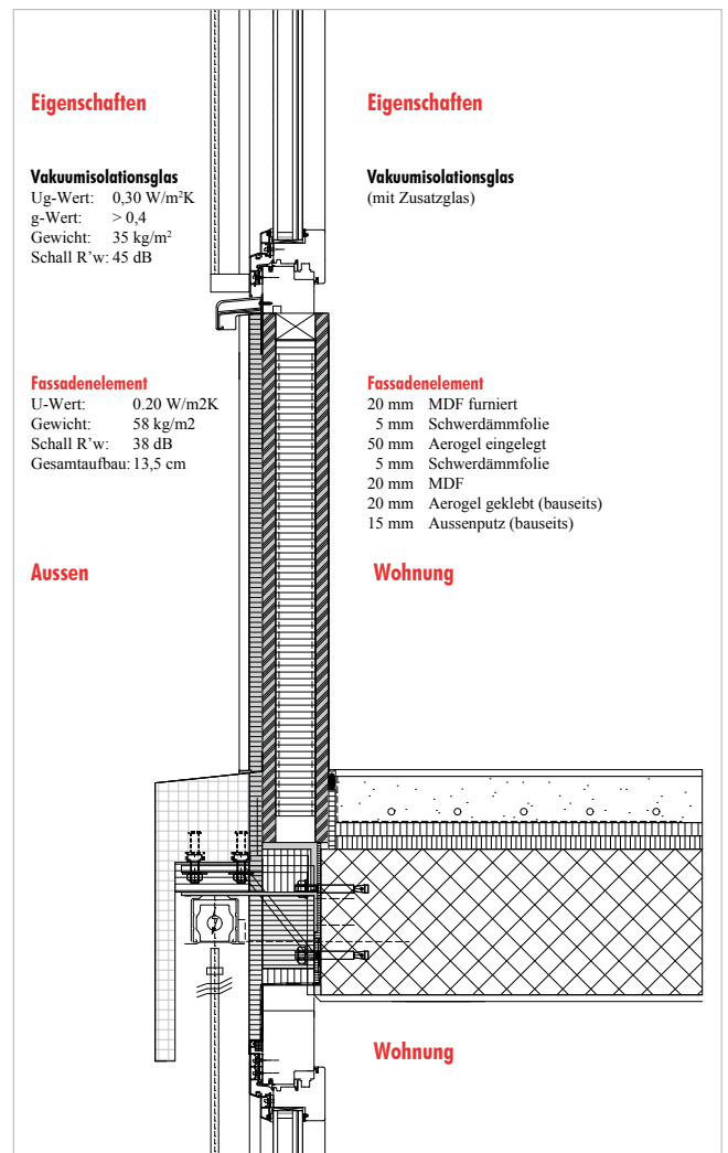
Abbildung 2: Detailschnitt Südfassade
