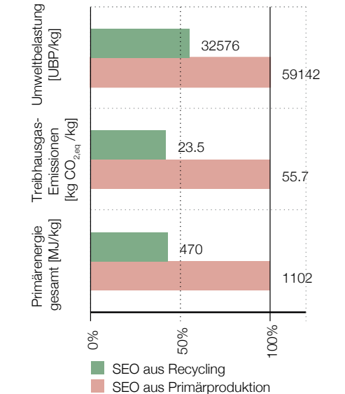
Abb. 5 Eine grobe Abschätzung der Ökobilanz (33) für die Primär- und Recyclingproduktion von SEO zeigt im Vergleich den deutlichen Vorteil von Recycling; jeweils skaliert auf 100% Primärproduktion.
