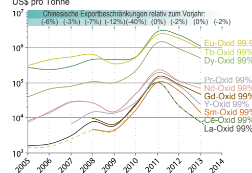
Abb. 7 Jährliche SEM-Preise (log. Skala) von Januar 2005 bis Januar 2014 (53). Deutlich erkennbar sind die Preisanstiege durch Chinesischen Exportrestriktionen und die Preisverfälle durch die Wirtschaftskrisen (2008, 2013/4).
