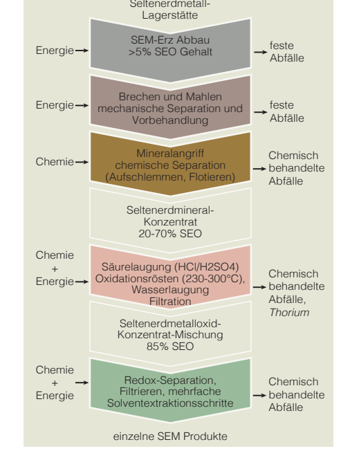
Abb. 6 Der Produktionsprozess von SEM von der Lagerstätte bis zu einzelnen SEO ist mit hohem Energieaufwand und grossen Umweltbelastungen verbunden (5,35).
