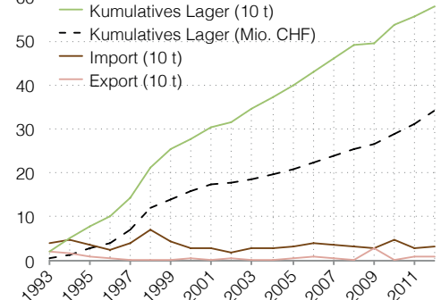
Abb. 8 Eine Hochrechnung der kumulativen SEO-Lager aus der Schweizer Import-Exportstatistik (15) liefert aufgrund versteckter Materialflüsse fragwürdige Ergebnisse.
